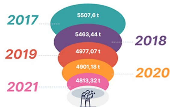
TERŠALŲ, IŠMESTŲ Į APLINKOS ORĄ IŠ STACIONARIŲ TARŠOS ŠALTINIŲ, KIEKIS KLAIPĖDOS REGIONE 2017-2021 M.
